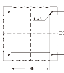
安裝孔 VFU01
